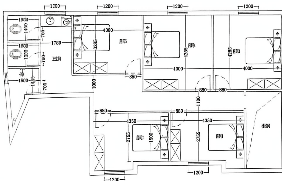
JL-2 驻地办平面图
